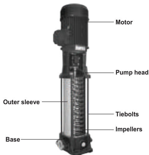
FIG. 3 LCR PUMP
